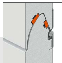
Isolasjons evne 60 mm. U=0,9 [ W/m^2K ]*
